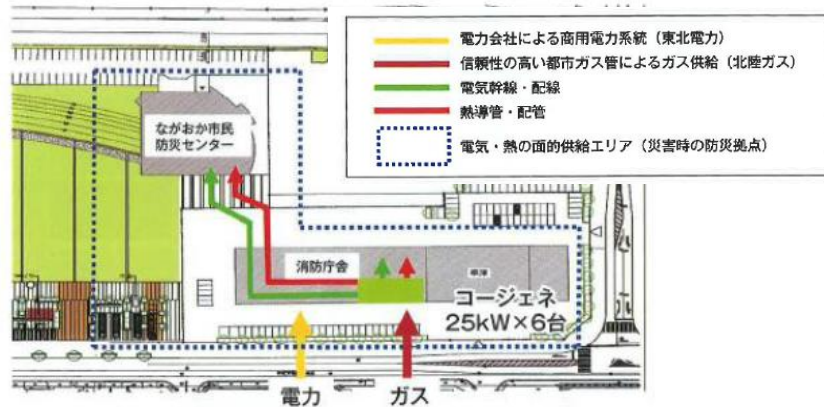
施設配置図
